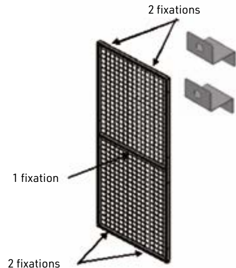
Modèle mural
